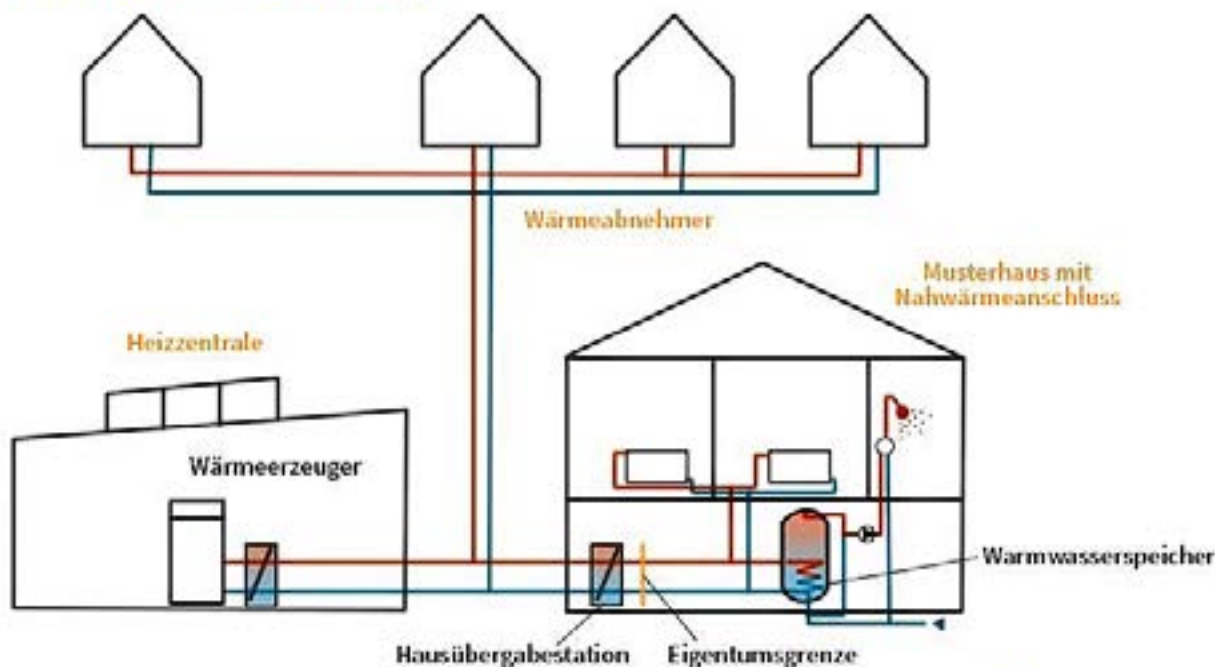
Bild 1: Prinzipielle Darstellung einer Nahwärmeversorgung Quelle: Kesselheld
